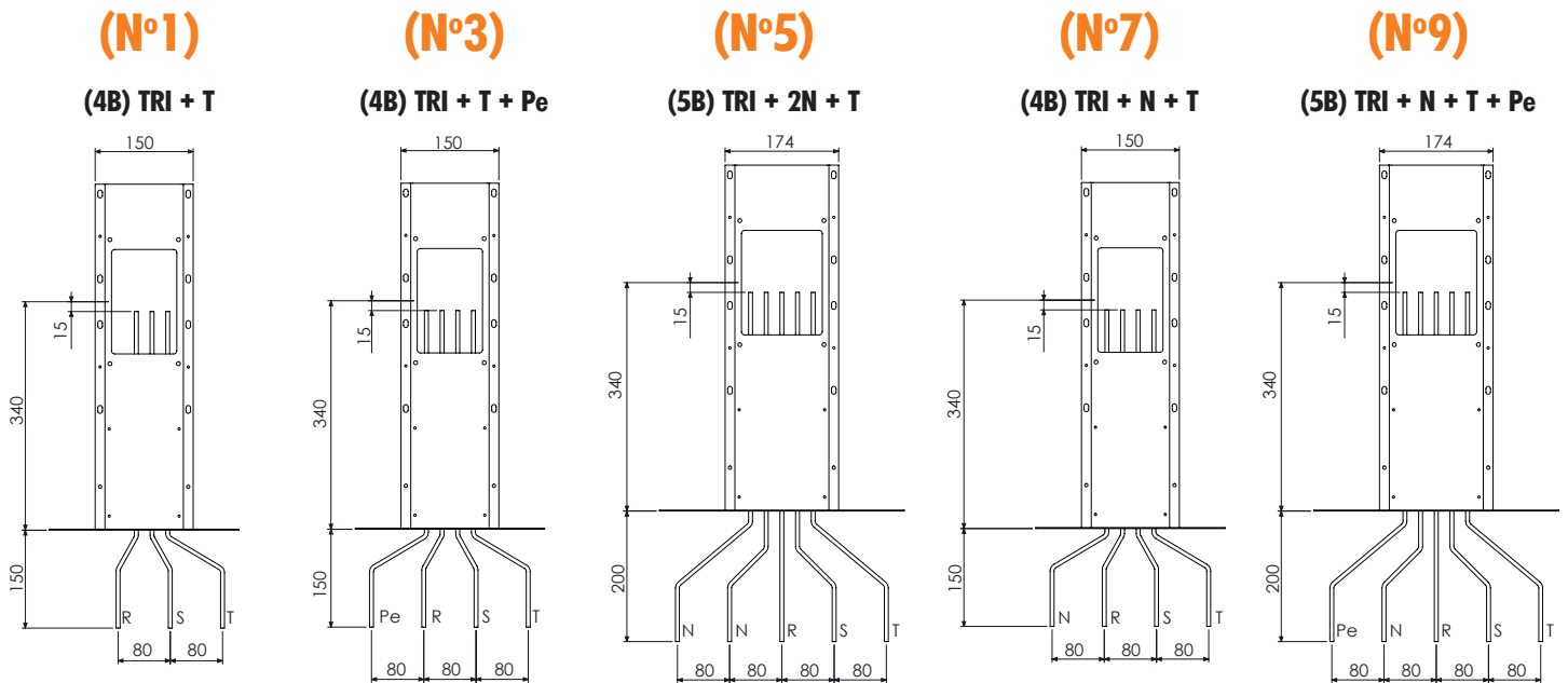
FLANGE UNIDAD TERMINAL (4B)
